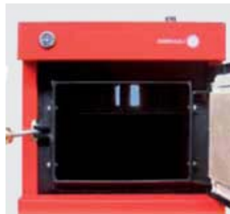
FRONTAL SUPERIOR EN QUE SE OBSERVA EL TERMÓMETRO DE CALDERA Y PASO DE HUMOS DE GRAN PASO PARA FACILITAR LAS TAREAS DE LIMPIEZA Y MANTENIMIENTO.
