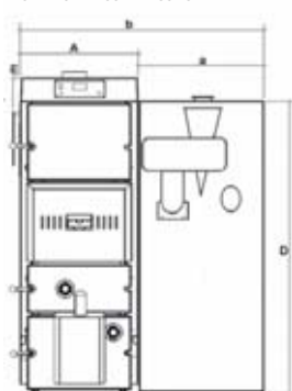
VISTA FRONTAL CON DEPÓSITO
